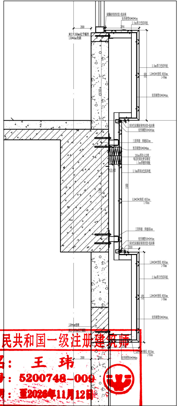
外墙铝单板详图
